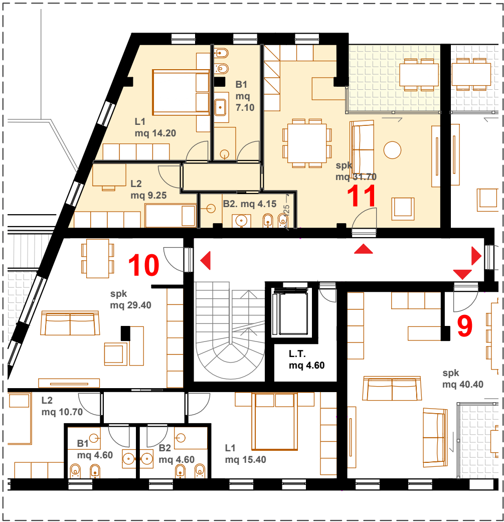
Planimetria piano secondo
