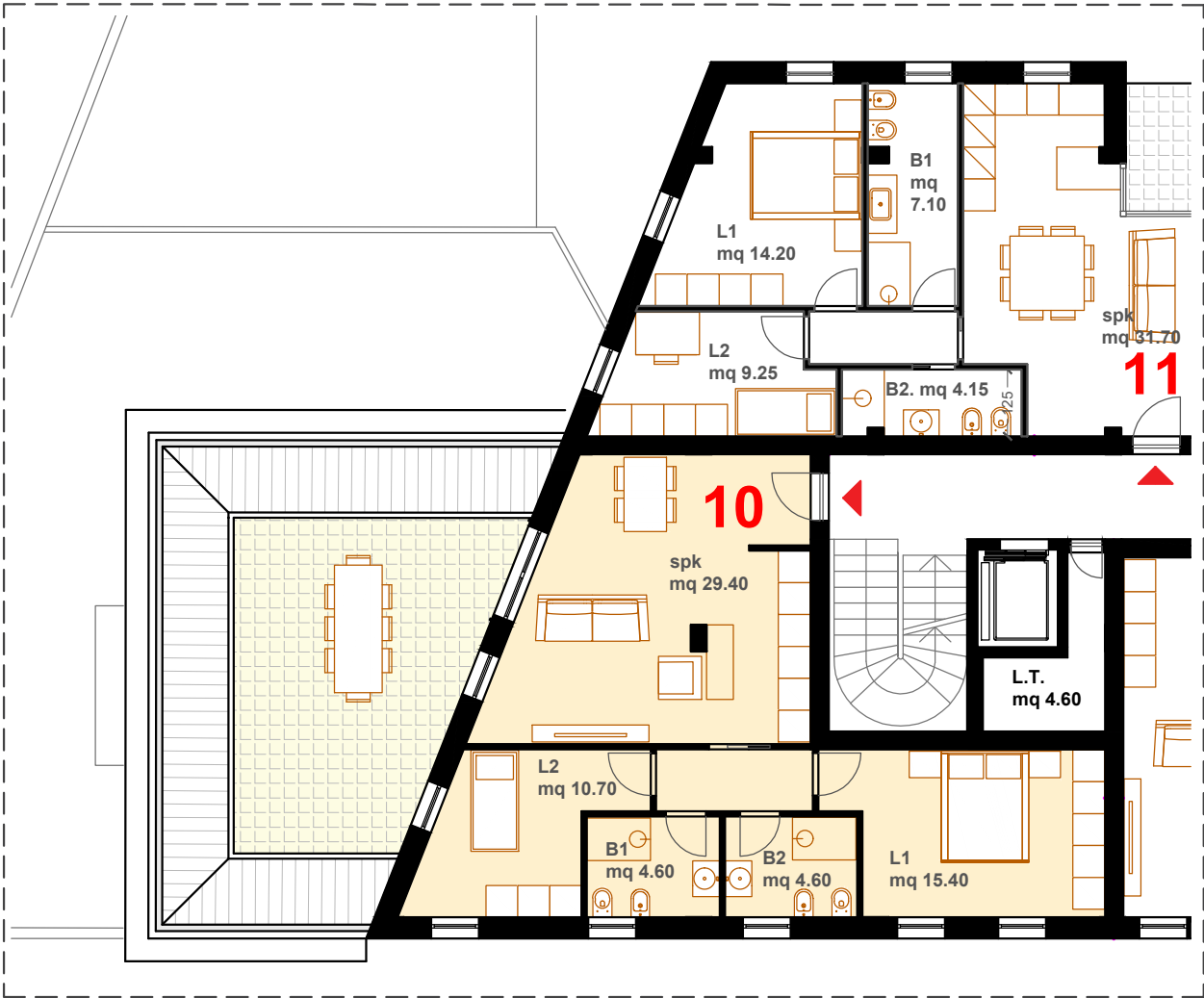
Planimetria piano secondo
