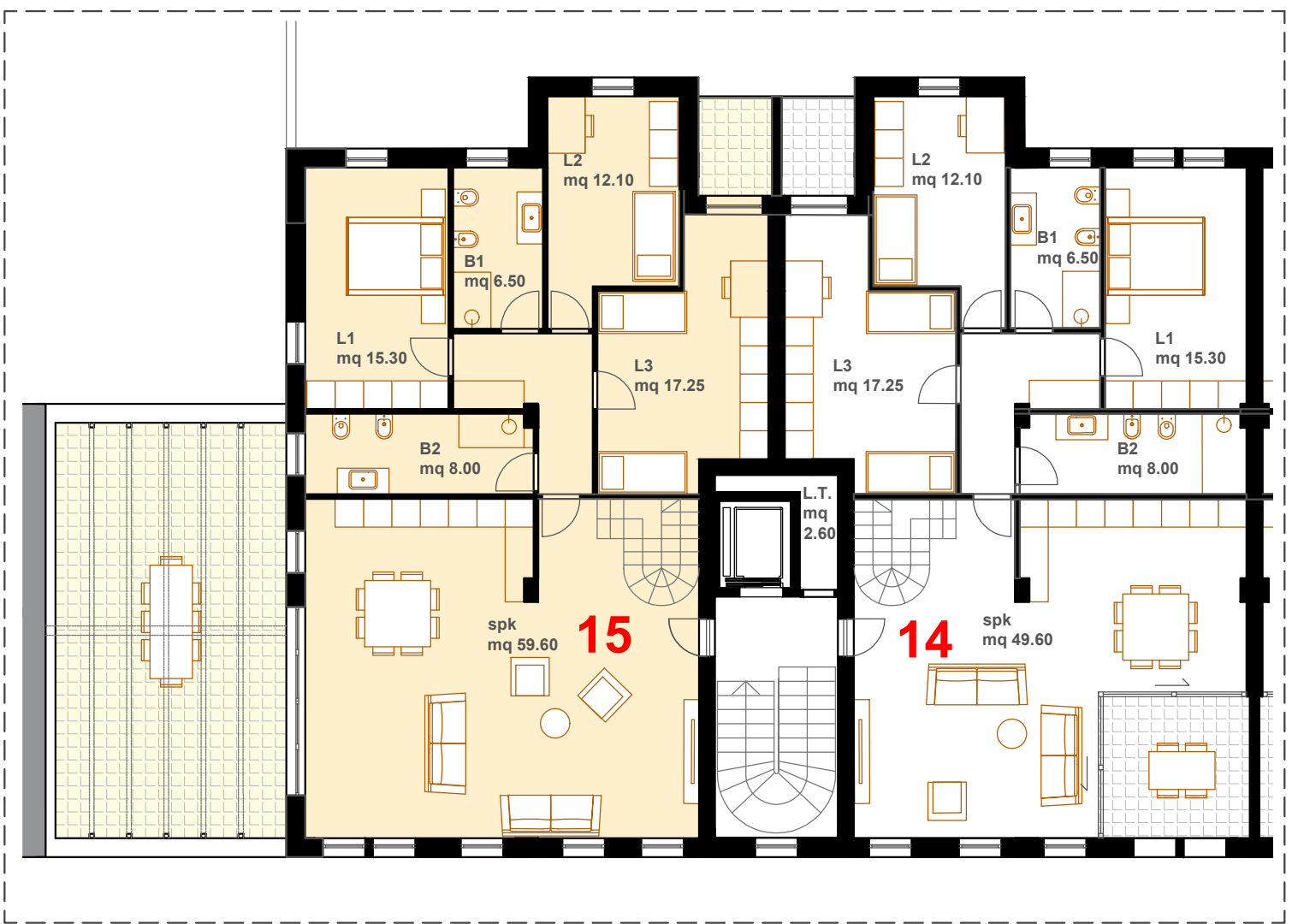
Planimetria piano secondo
