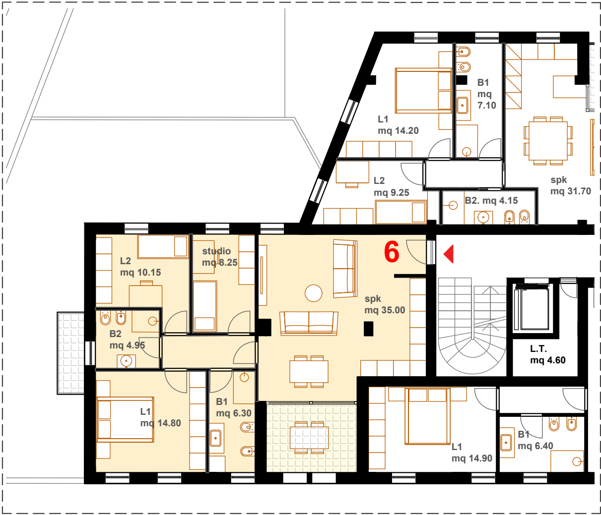
Planimetria piano primo
