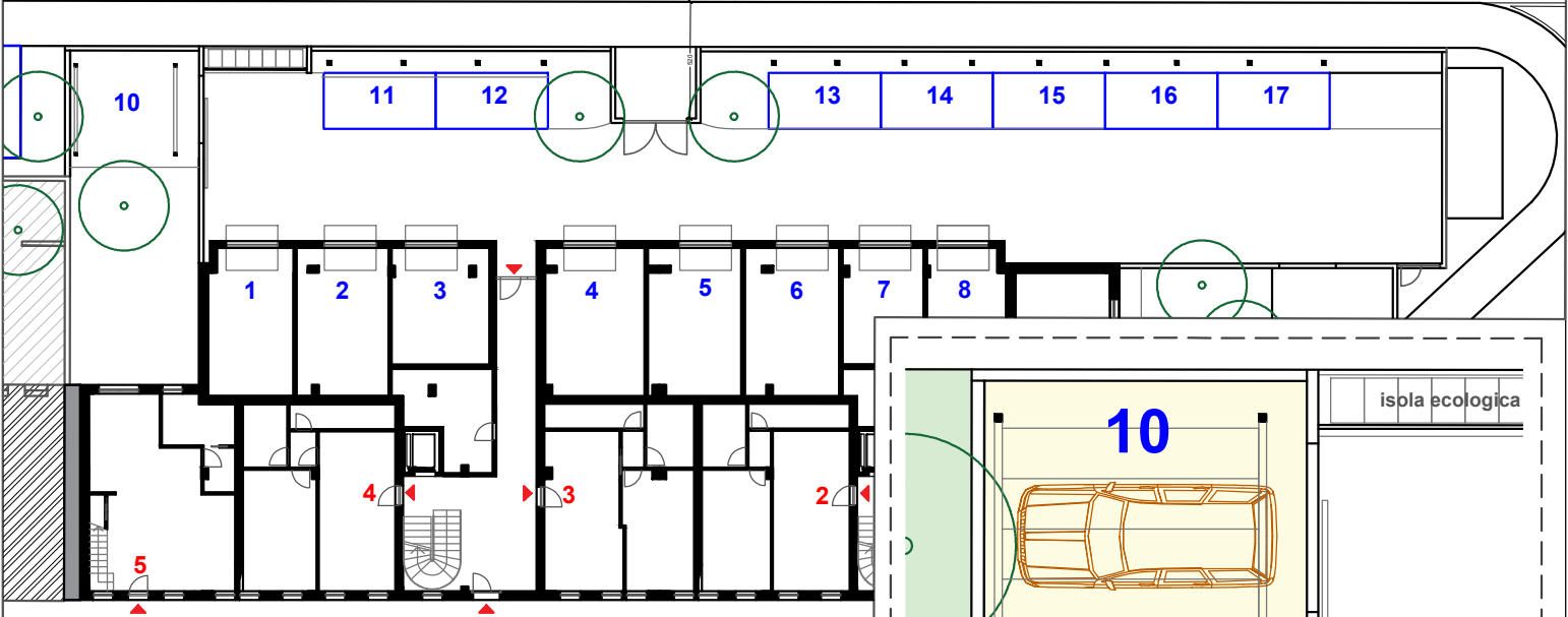
Planimetria piano terra e primo
